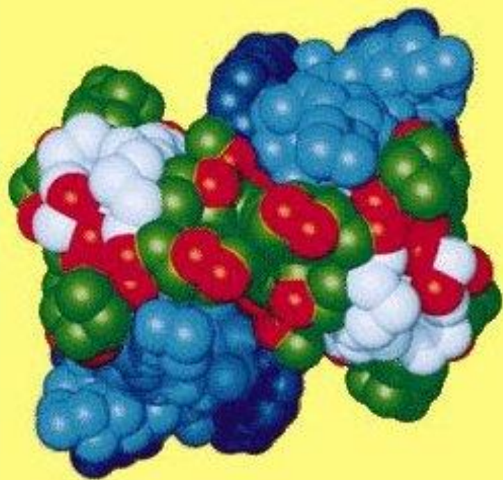
Histone Octamer
